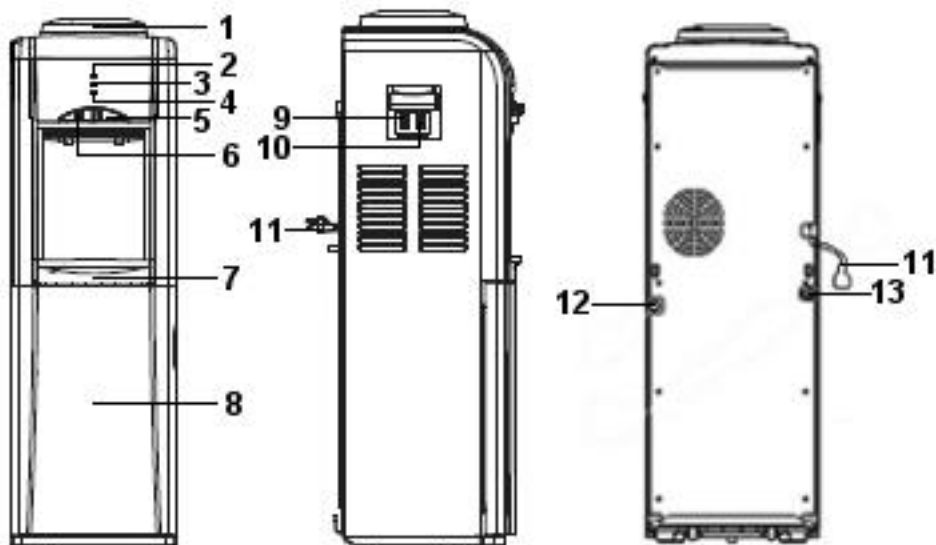
Рис.1. Схема аппарата V802CE, V802CES
